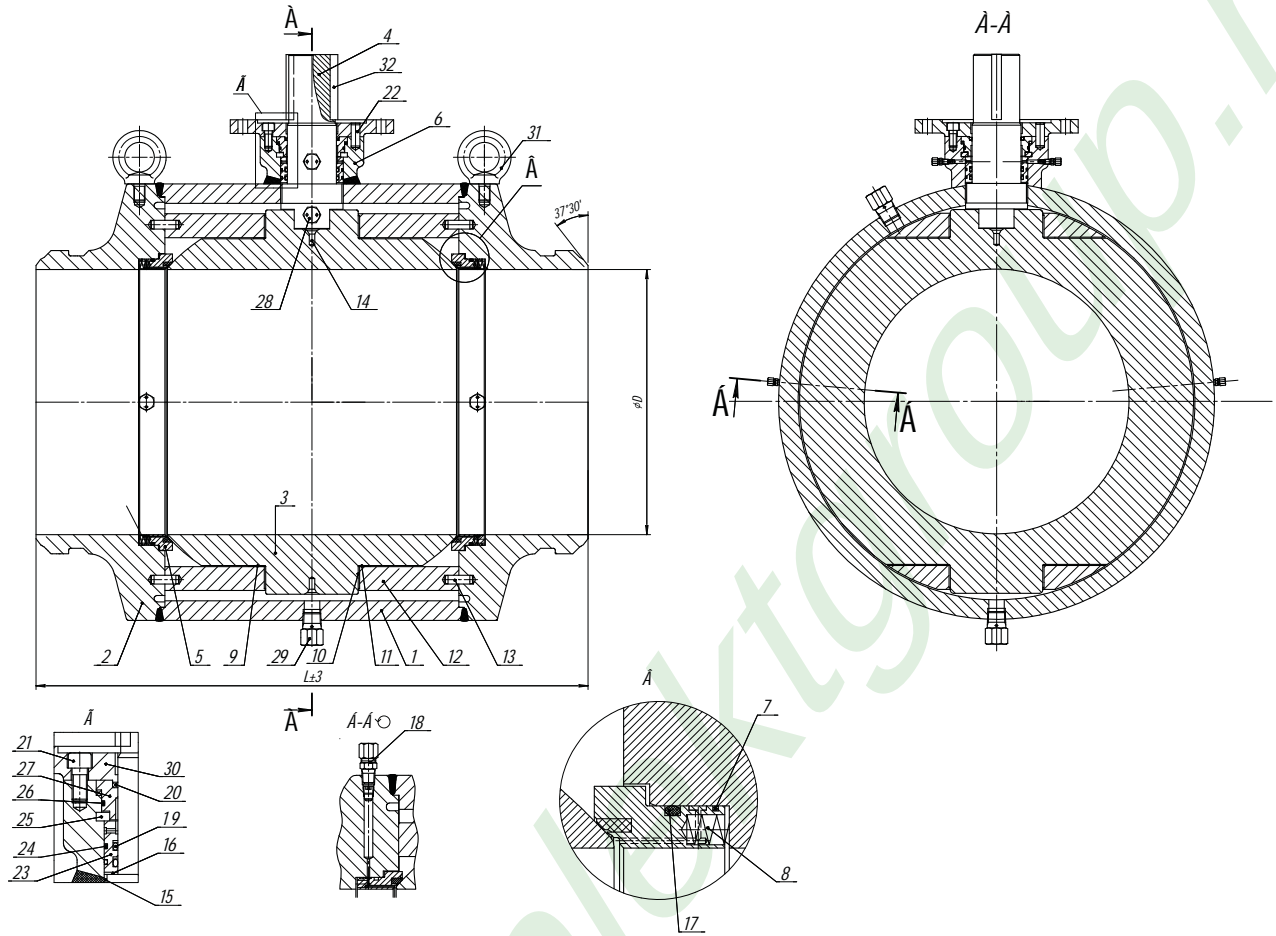
DN 350–1200 (14 серия)
