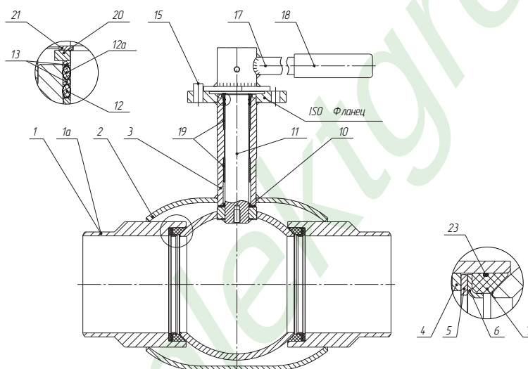
DN 100–400 (15 серия)
