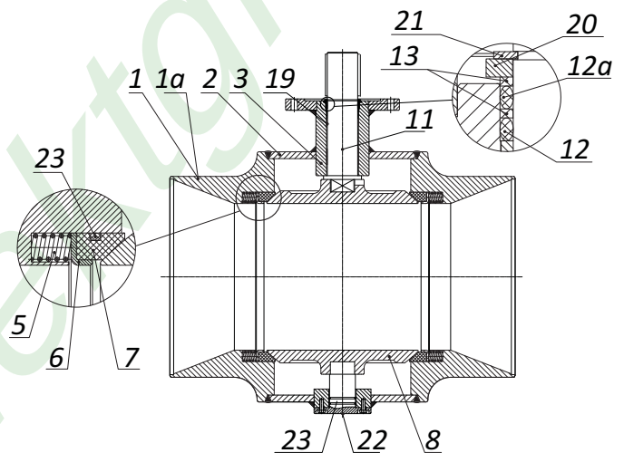
DN 400–600 (11 серия)
