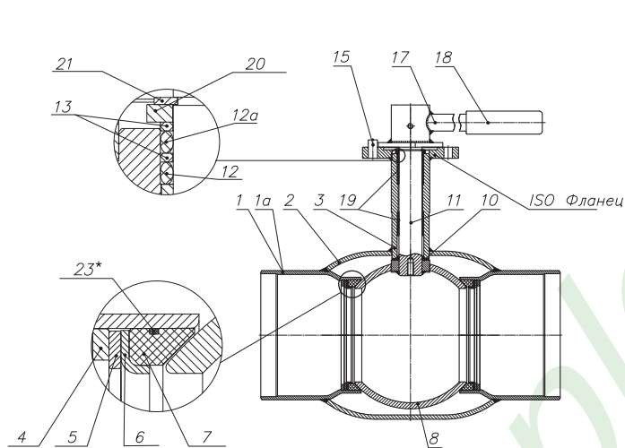
DN 125–500 (12 серия)
